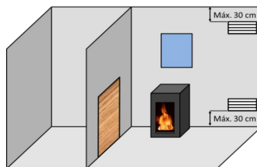
Figura nº6 - Schéma indicatif pour les grilles de ventilation
