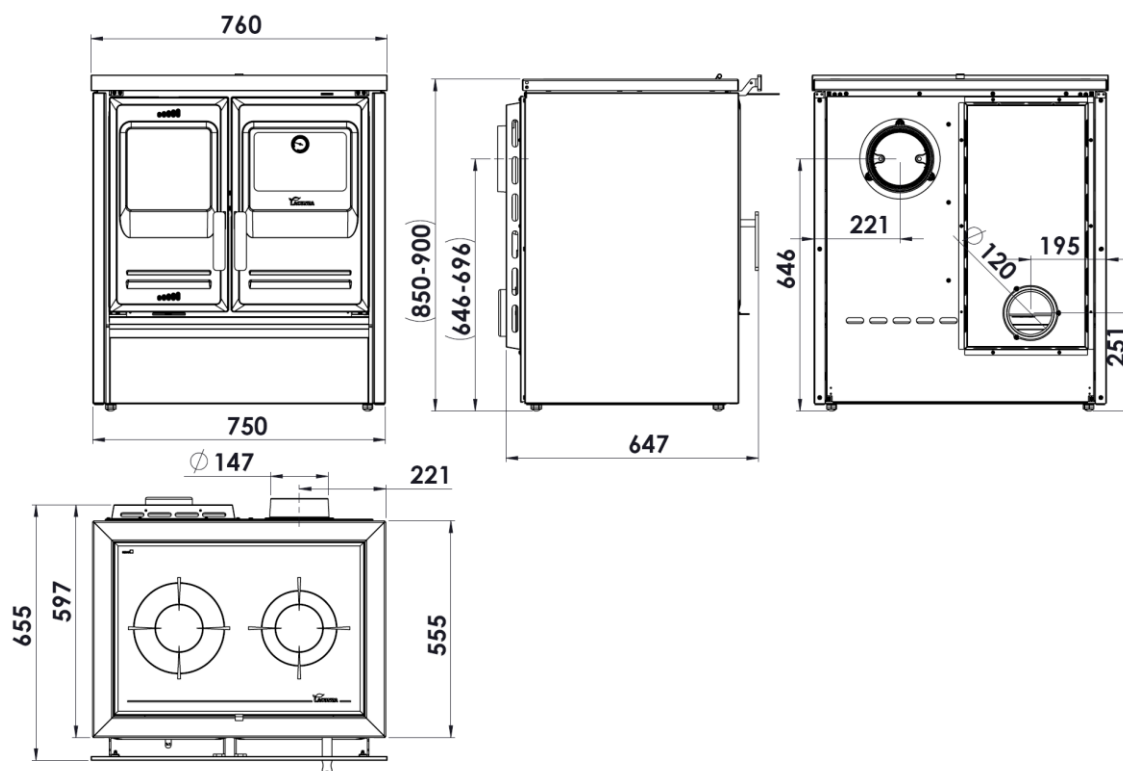
Figura n°2 - Dimensions en mm de l'appareil ETNA 5T TOP
